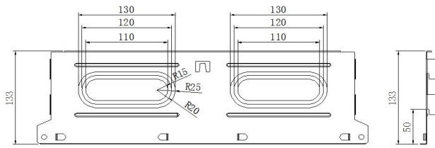
挂板切面图
