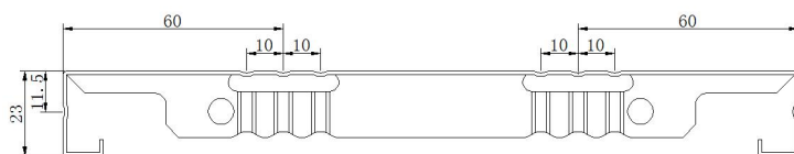
搁板切面图
